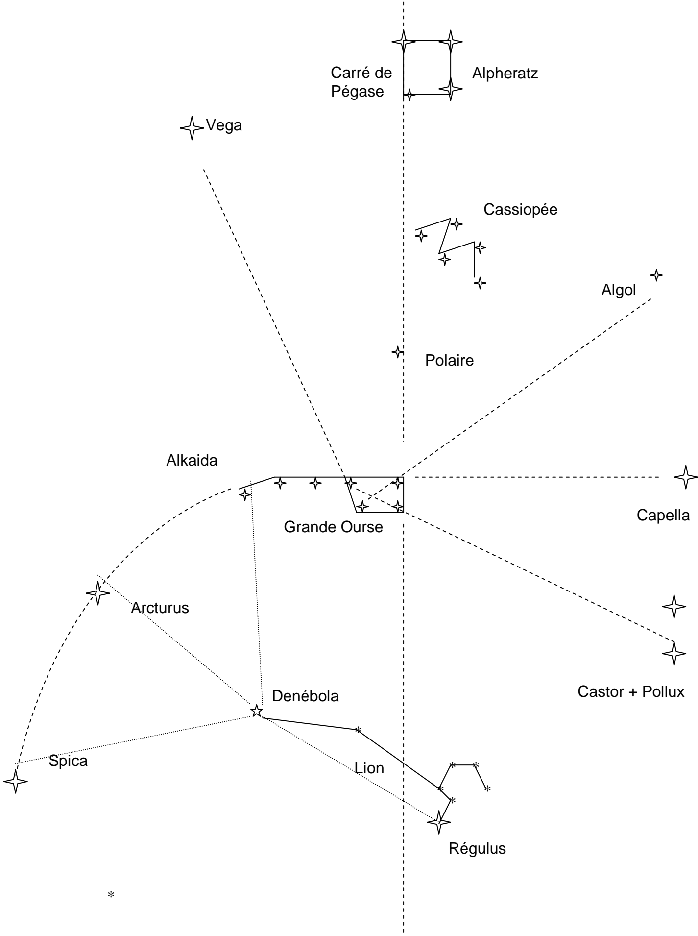
Alignements en partant de la Grande Ourse, étoiles du printemps
